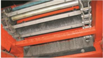
配有链条清扫装置，防止融雪剂带入货厢对其产生腐蚀
